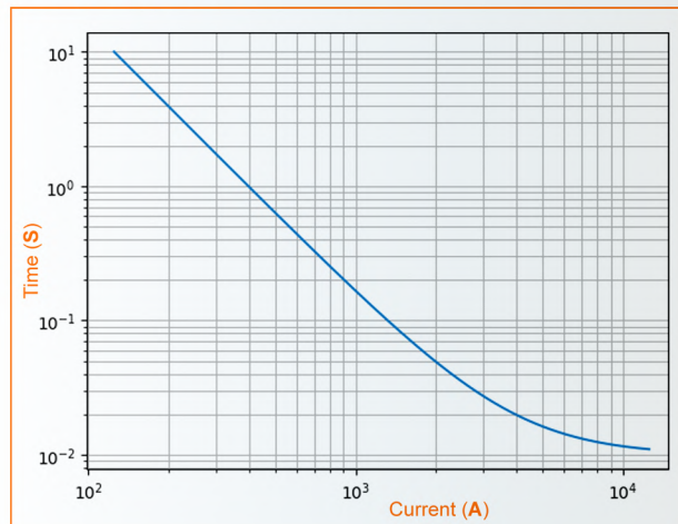
Model NH00-125A
